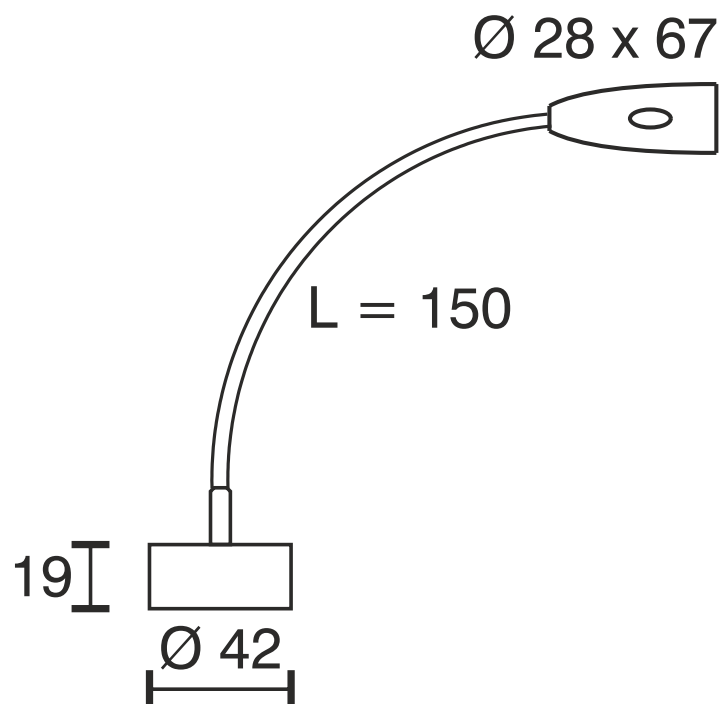
Leuchtenkopf Ø 28 x 67 mm
